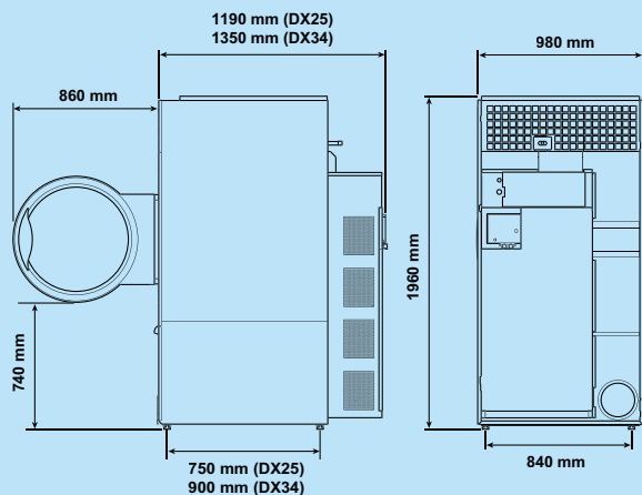
Seitenansicht DX 25 34
